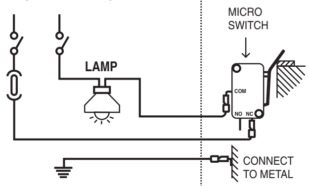
230 VAC (o 115 VAC) ALIMENTAZIONE LAMPADARIO
